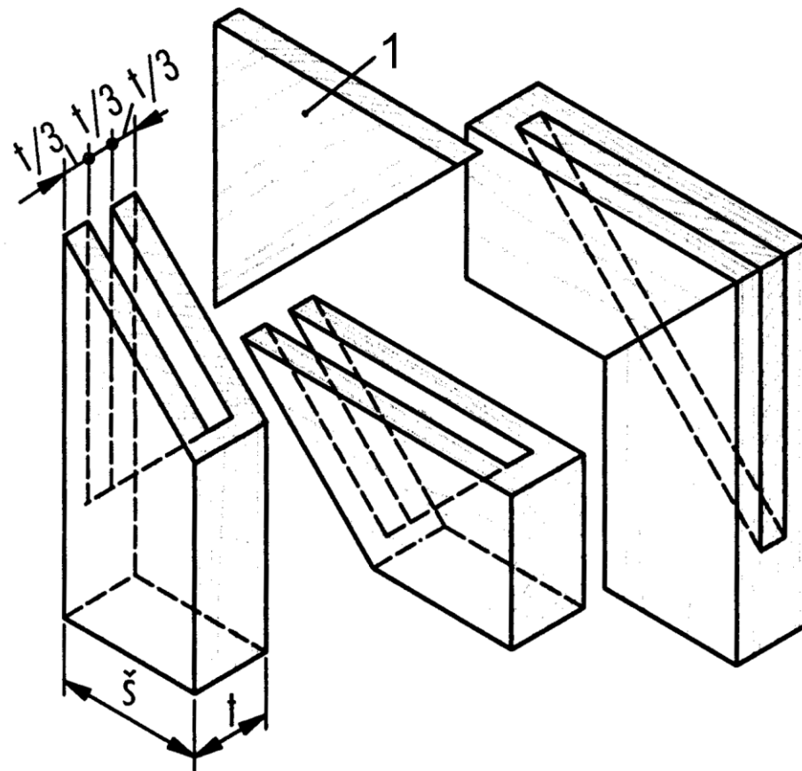
Spoj na pokos s vlepéným cudzím perom (1) z masívneho dreva
