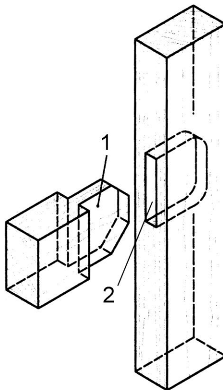
Čap a dlab – stredový spoj (1 – čap nepriebežný; 2 – dlab)
