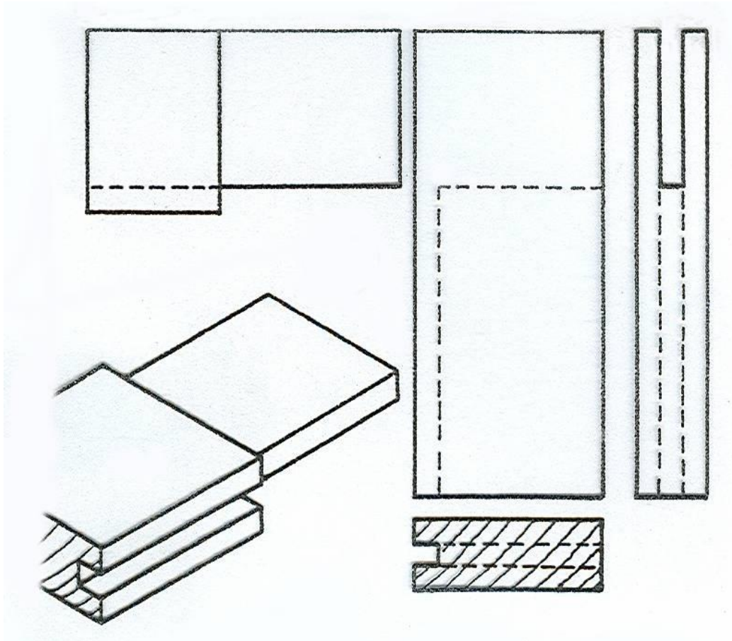
Čap a rozčap s drážkou s hrúbkou 1/3
