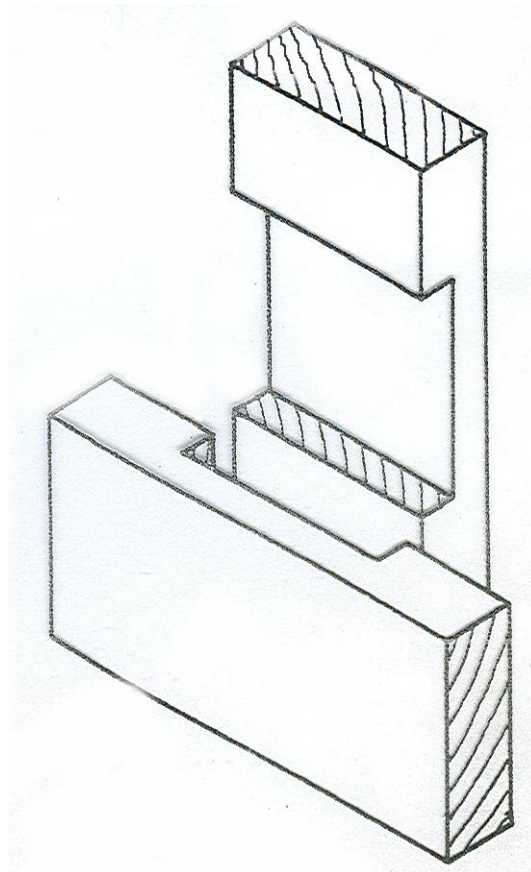
Preplatovanie – krížový spoj
