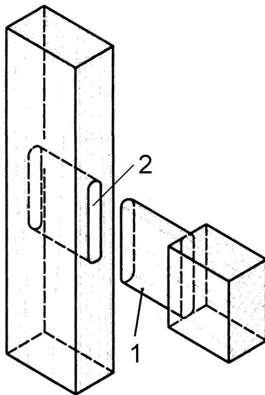
Čap a dlab – stredový spoj (1 – čap priebežný; 2 – dlab)
