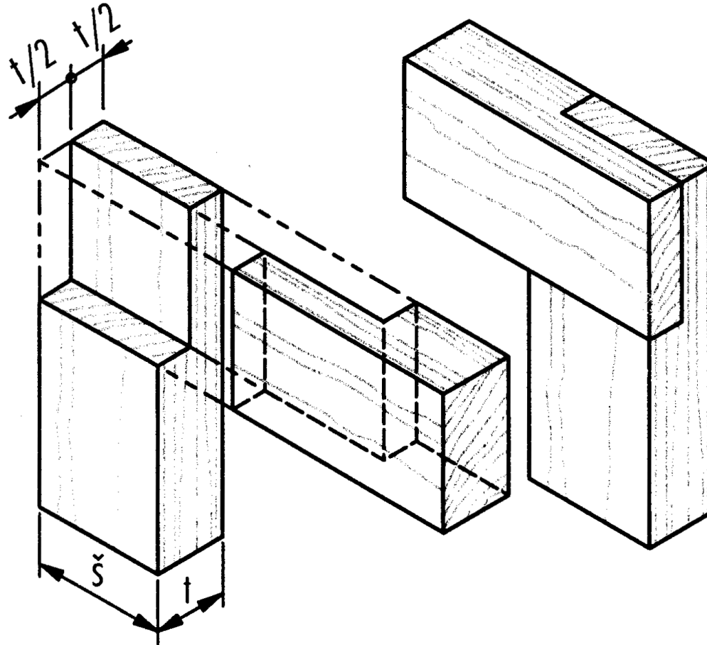
Preplatovanie – rohový spoj
