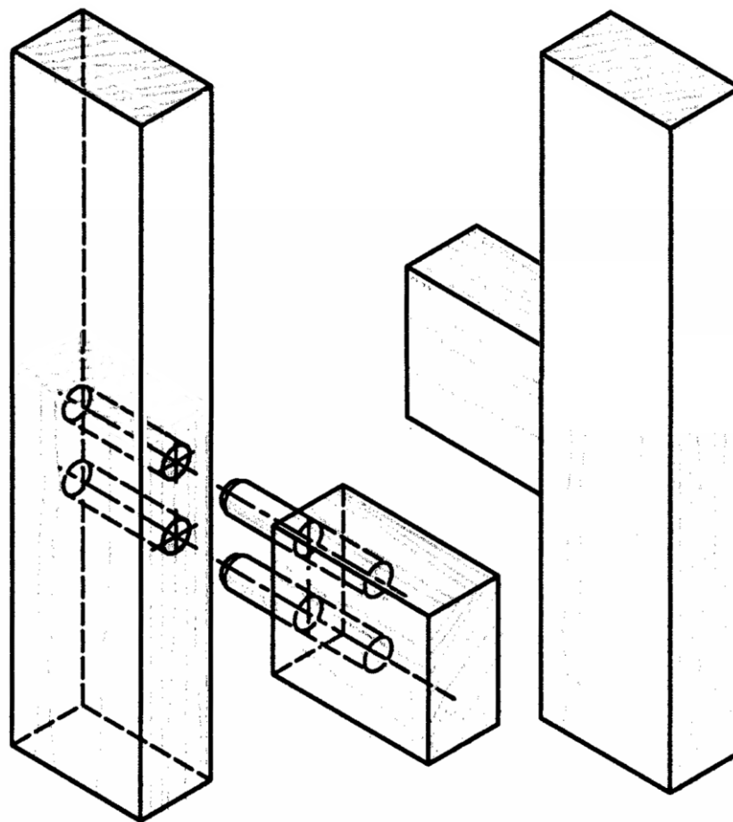
Spoj na kolíky – na tupo, stredový
