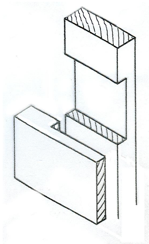
Preplatovanie – stredový spoj
