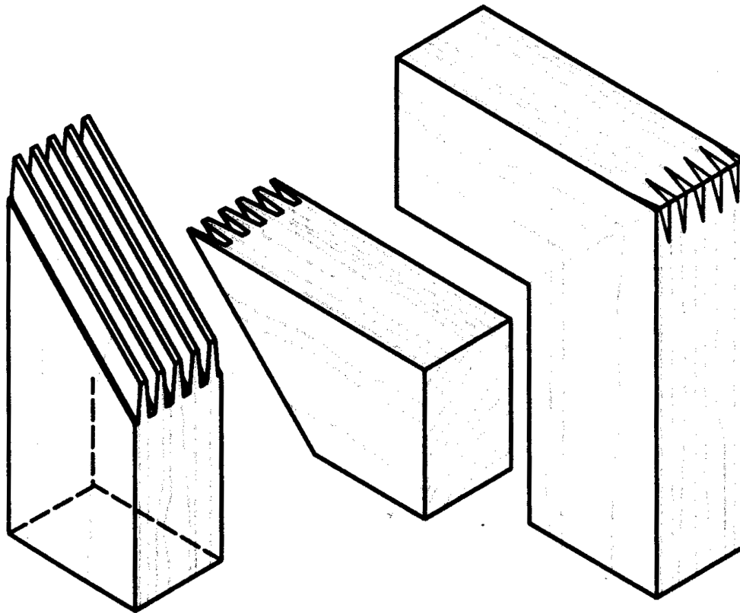
Spoj na pokos na klinové ozuby
